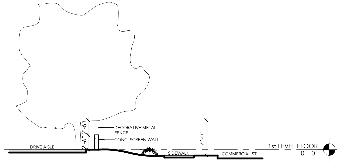
5 SITE SECTION SCALE: 1/8" = 1'-0"
