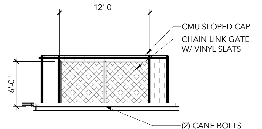
2 TRASH - WEST ELEVATION SCALE: 1/8" = 1'-0"
