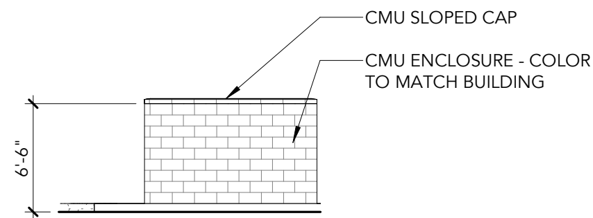
3 TRASH - SOUTH ELEVATION SCALE: 1/8" = 1'-0"
