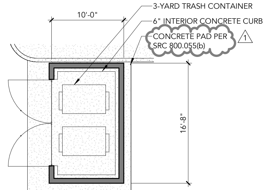
1 TRASH ENCLOSURE SCALE: 1/8" = 1'-0"
