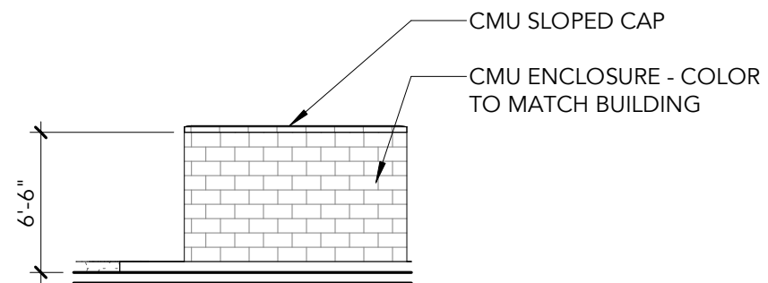
4 TRASH - SOUTH ELEVATION SCALE: 1/8" = 1'-0"
