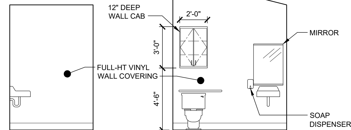
H TOILET - 104
