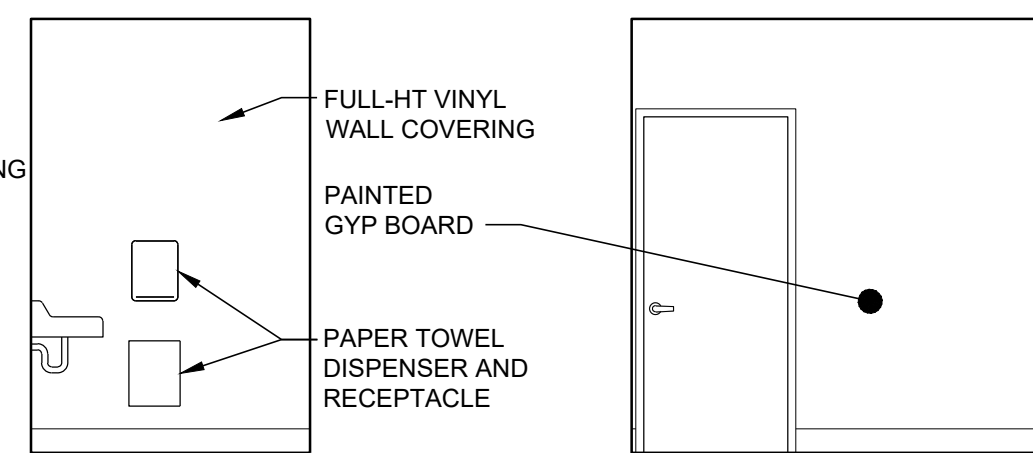
G TOILET - 104
