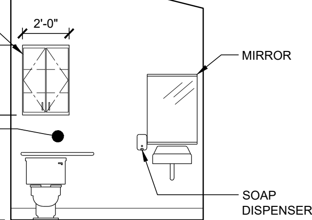
K TOILET - 203
