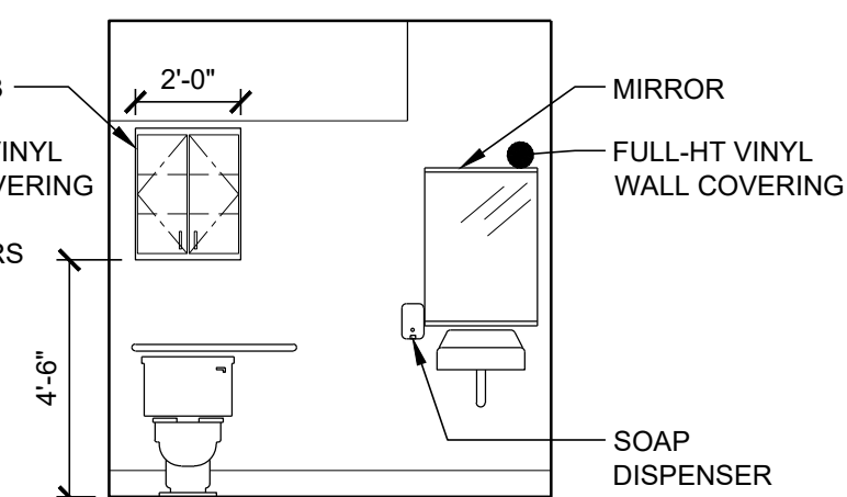
F TOILET - 104
