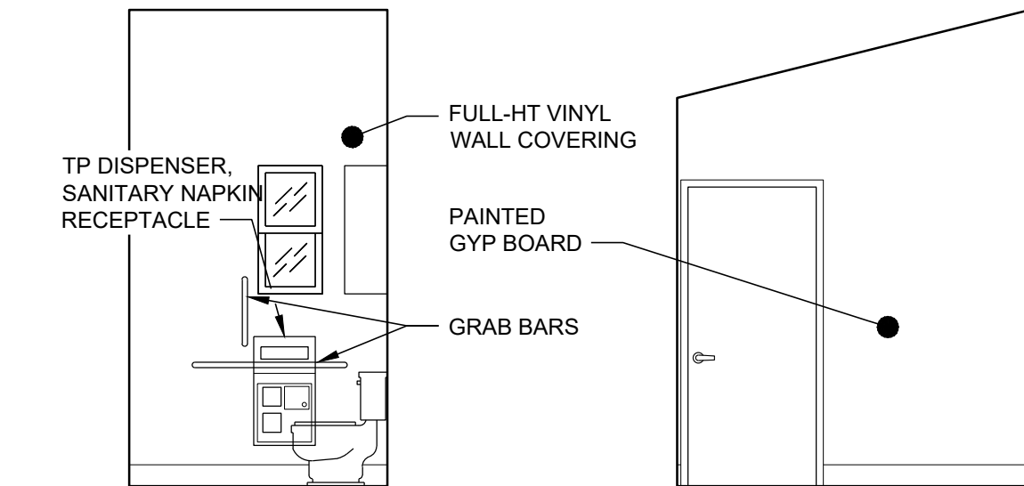
L TOILET - 203
