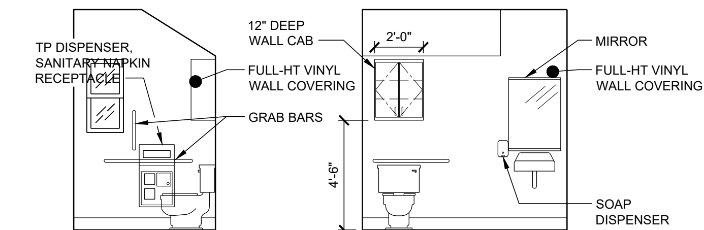
E TOILET - 104
