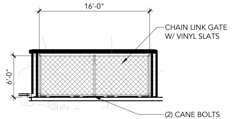
2 TRASH - WEST ELEVATION SCALE: 1/8" = 1'-0"
