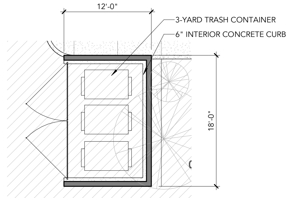
1 TRASH ENCLOSURE SCALE: 1/8" = 1'-0"
