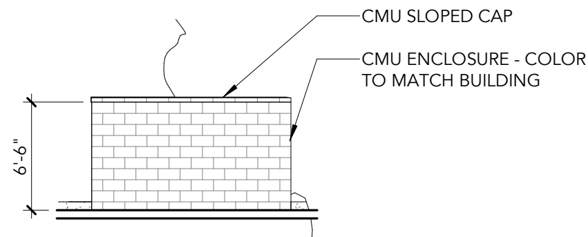
4 TRASH - SOUTH ELEVATION SCALE: 1/8" = 1'-0"
