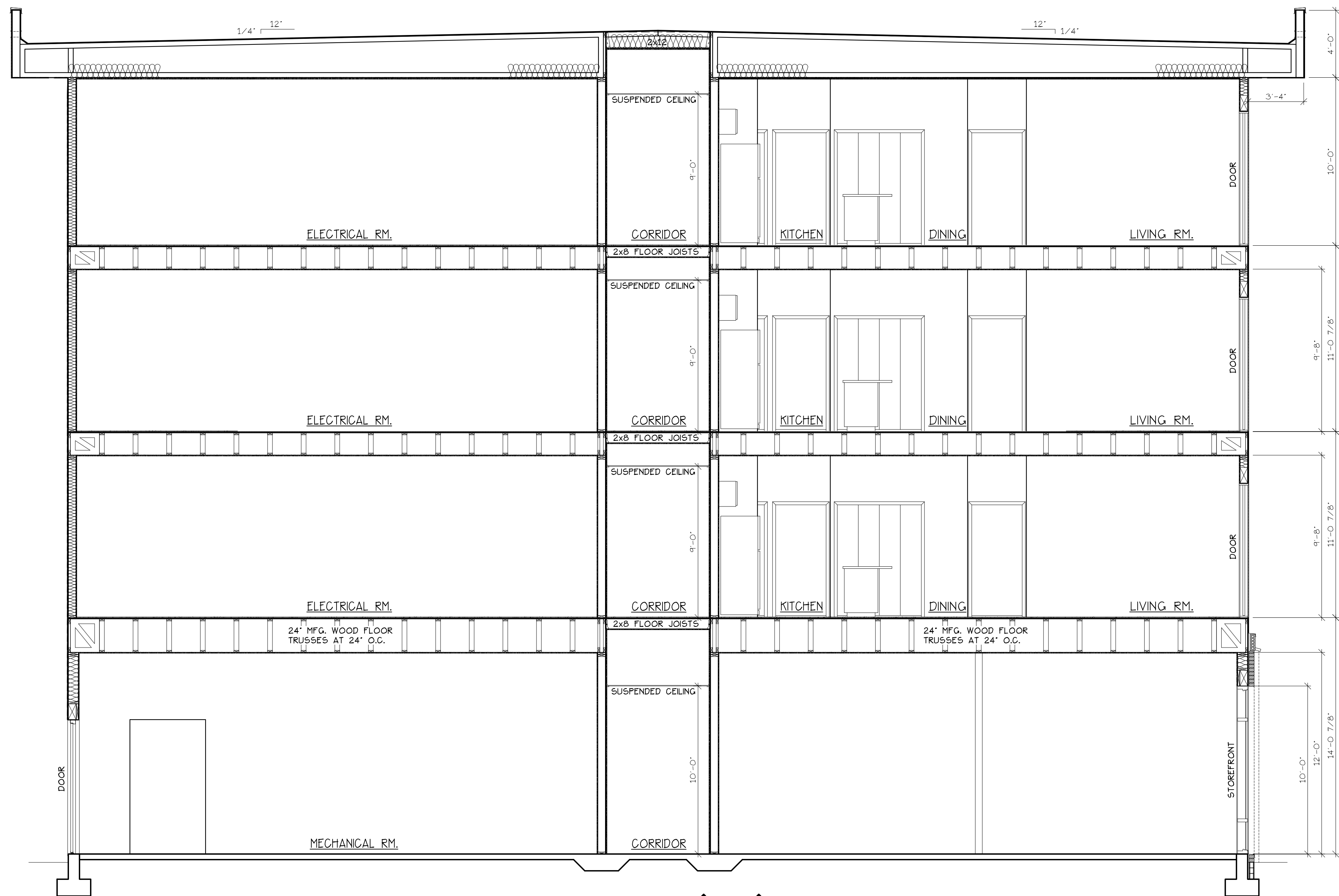
SECTION C-C SCALE: 1/4" = 1'-0" A1.31 THRU A1.37
