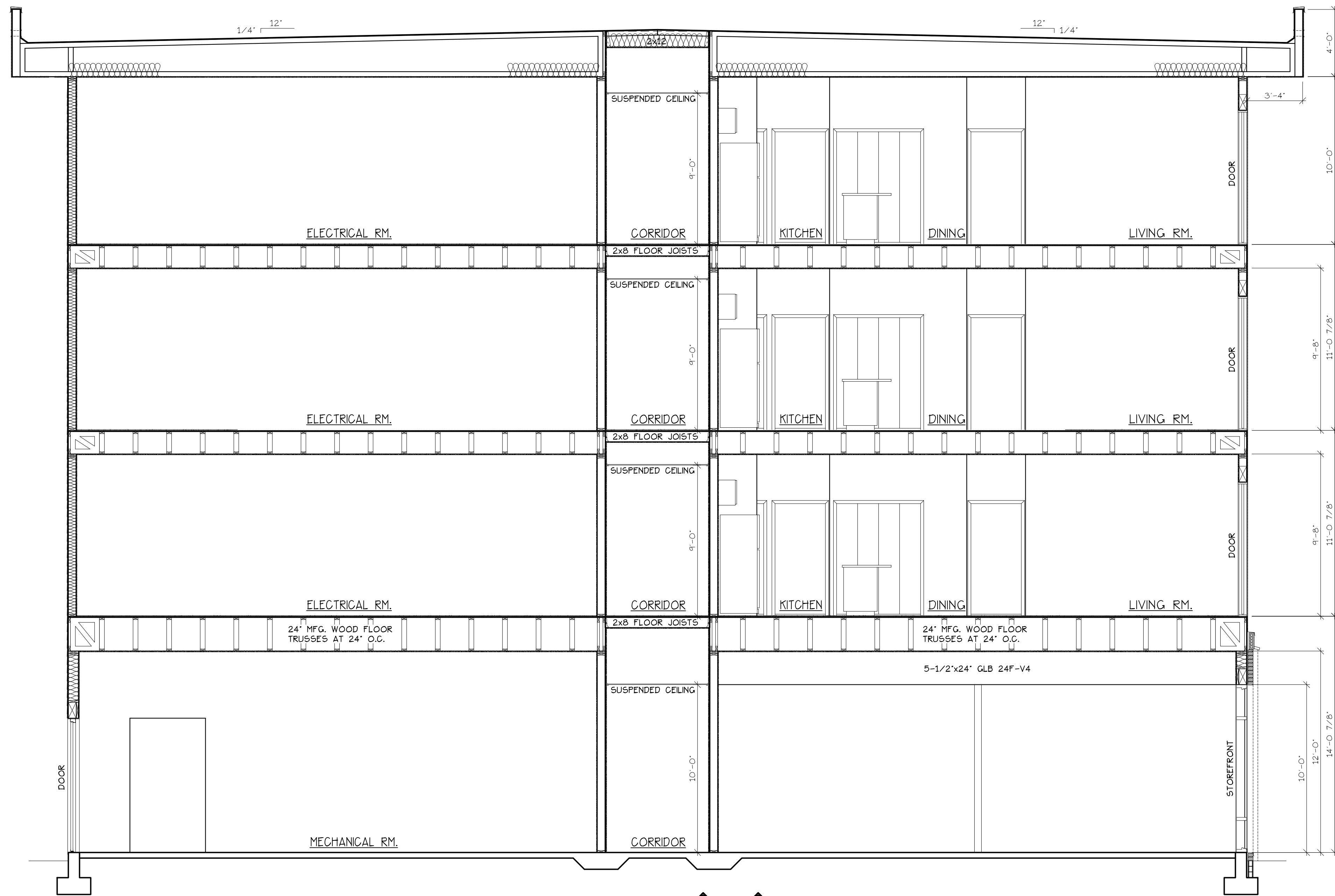
SECTION C-C SCALE: 1/4" = 1'-0"
