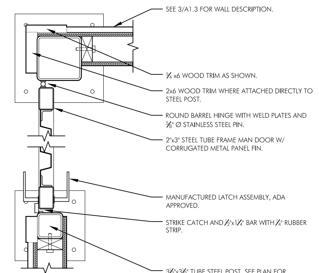
3 TRASH ENCLOSURE MAN DOOR DETAIL
